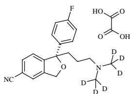
R-(-)-Citalopram-d 6 Oxalate
