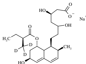
Pravastatin-d 3
