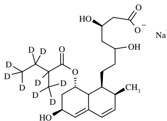
Pravastatin-d 9 (racemic)
