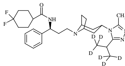
Maraviroc-d6
