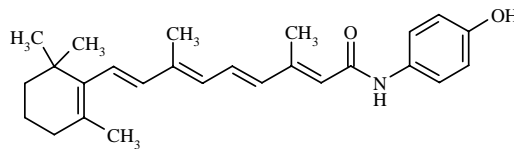
Fenretinide
