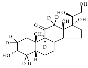
Allotetrahydrocortisol-d 7
