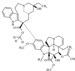
Vinblastine-d 3
