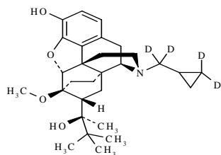
Buprenorphine-d 4
